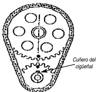
Figura 3 Estándar
