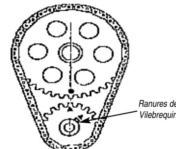
Figure 7 4° Avancé
