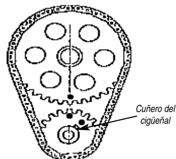
Figura 6 Estándar
