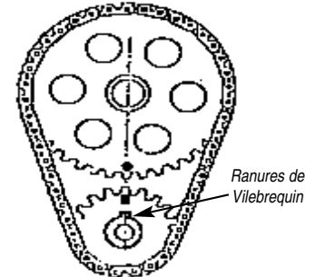
Figure 5 4° Retard
