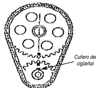
Figura 5 4° Retardado
