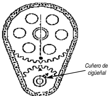
Figura 7 4° Avanzado
