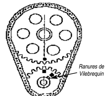
Figure 8 4° Retard
