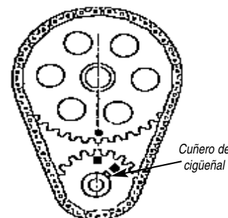
Figura 8 4° Retardado
